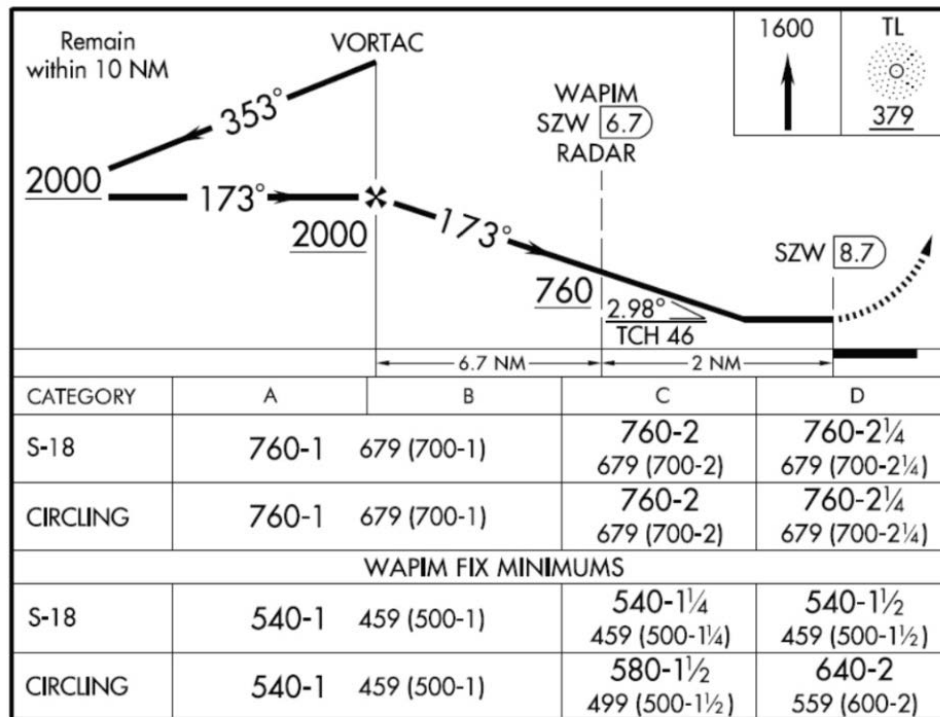
Figure 16.8. KTLH VOR 18.
