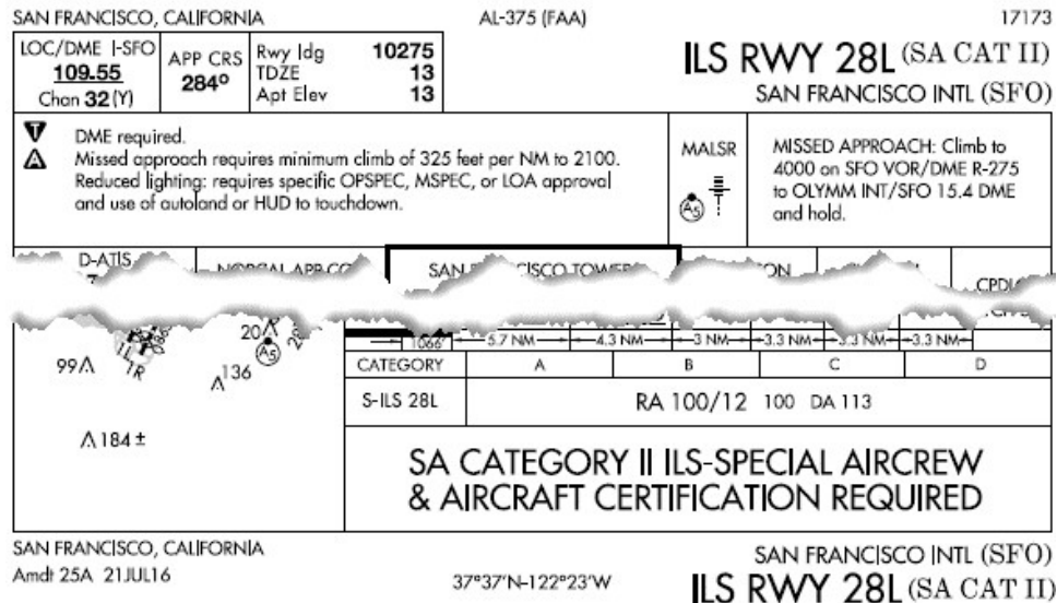
Figure 17.4. SA CAT II ILS Approach.
